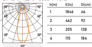
DP-SMP-AL10 3000K 90Ra
