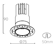
DP-RMSA-ER10/12(TL) Trimless
