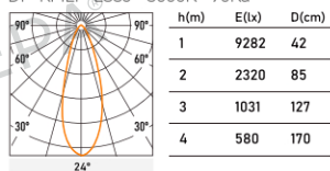
DP-RMLP-LS35 3000K 90Ra
