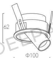
DP-RMSP-MC10 Fixed
