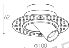
DP-RMSP-MC10(TL) Trimless
