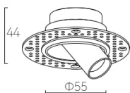
DP-RMSP-MC5(TL) Trimless
