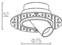
DP-RMSP-MC7(TL) Trimless
