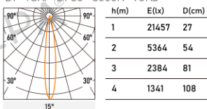
DP-TSRP-OP30 3000K 95Ra
